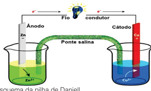
Esquema da pilha de Daniell.
